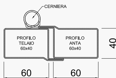
telaio B.TL
