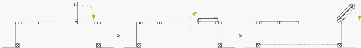
D 4 ante | anta principale a spingere | 2 dx e 2 sx
