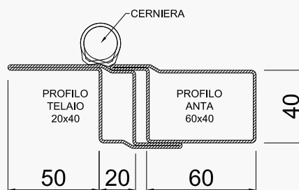
telaio D.TL
