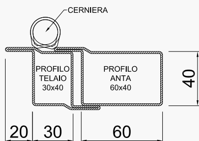
telaio A.TL
